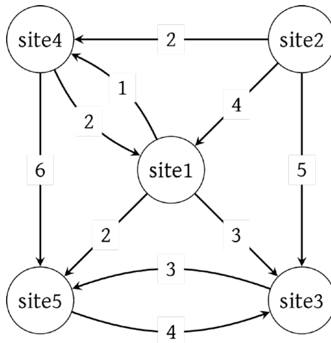
FIGURE 1. GRAPHE AVEC 5 SITES
